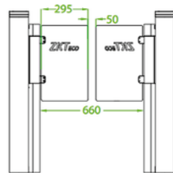
Barrera peatonal de medio cuerpo
